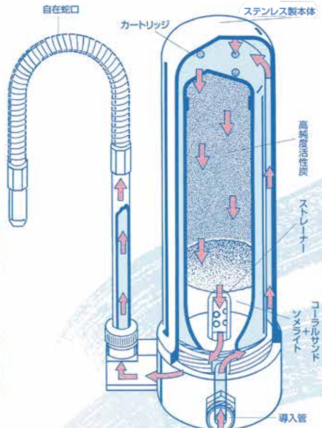
《アクアピュア S の構造図》
